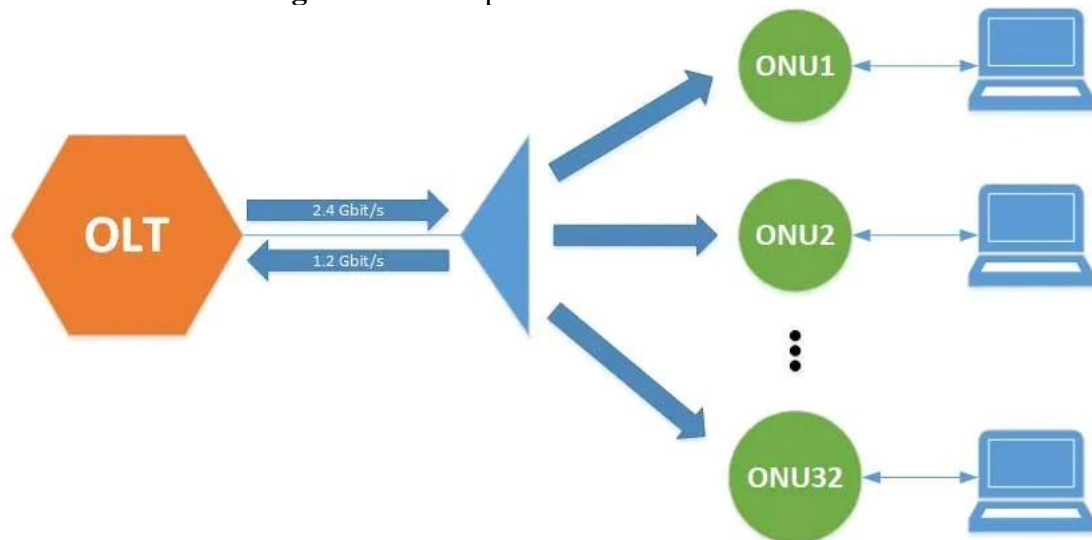
Figura 2.6: Componentes de una red GPON.
