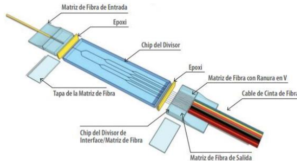
Figura 2.12: Técnica PLC
