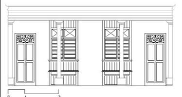
DETALLE 2- Ventanas de chazas y antepecho listonado, puerta con celosías superiores ornamentadas
