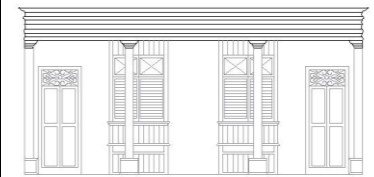
DETALLE 1- Cornisas y capiteles moldurados
