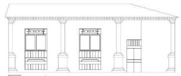
DETALLE 2- Ventanas abatibles con celosía superior ornamentada y balcones listonados
