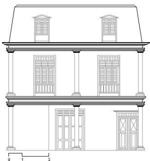
DETALLE 1- Cornisas y capiteles moldurados
