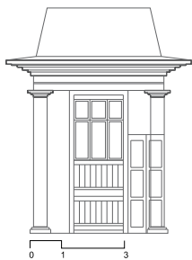
Detalle 1- Cornisas molduradas
